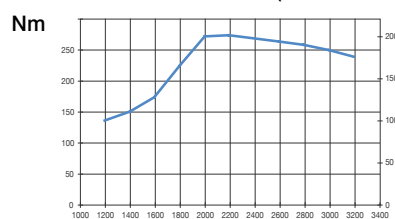
Drehmoment in Nm (Kurbelwelle)
